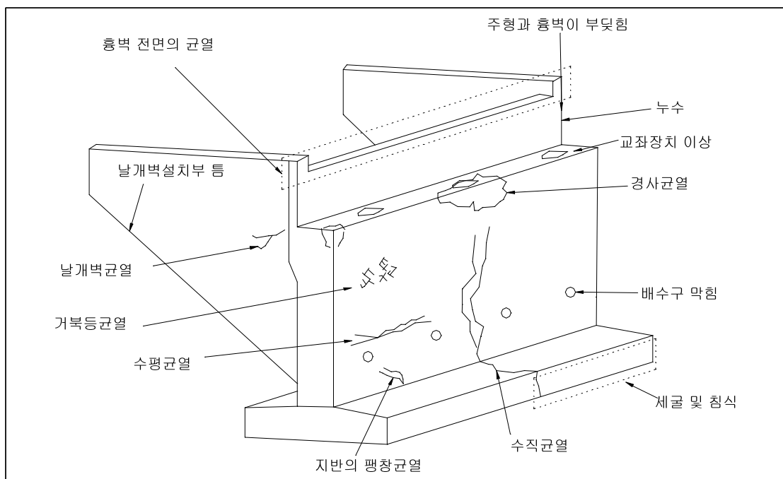
【그림 3.2.9】 교대의 점검부위
