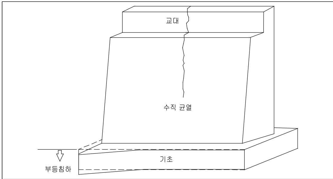
【그림 3.2.8】 부등침하로 인한 교대의 수직균열
