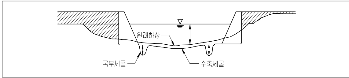
【그림 3.2.12】 수축세굴과 국부세굴
