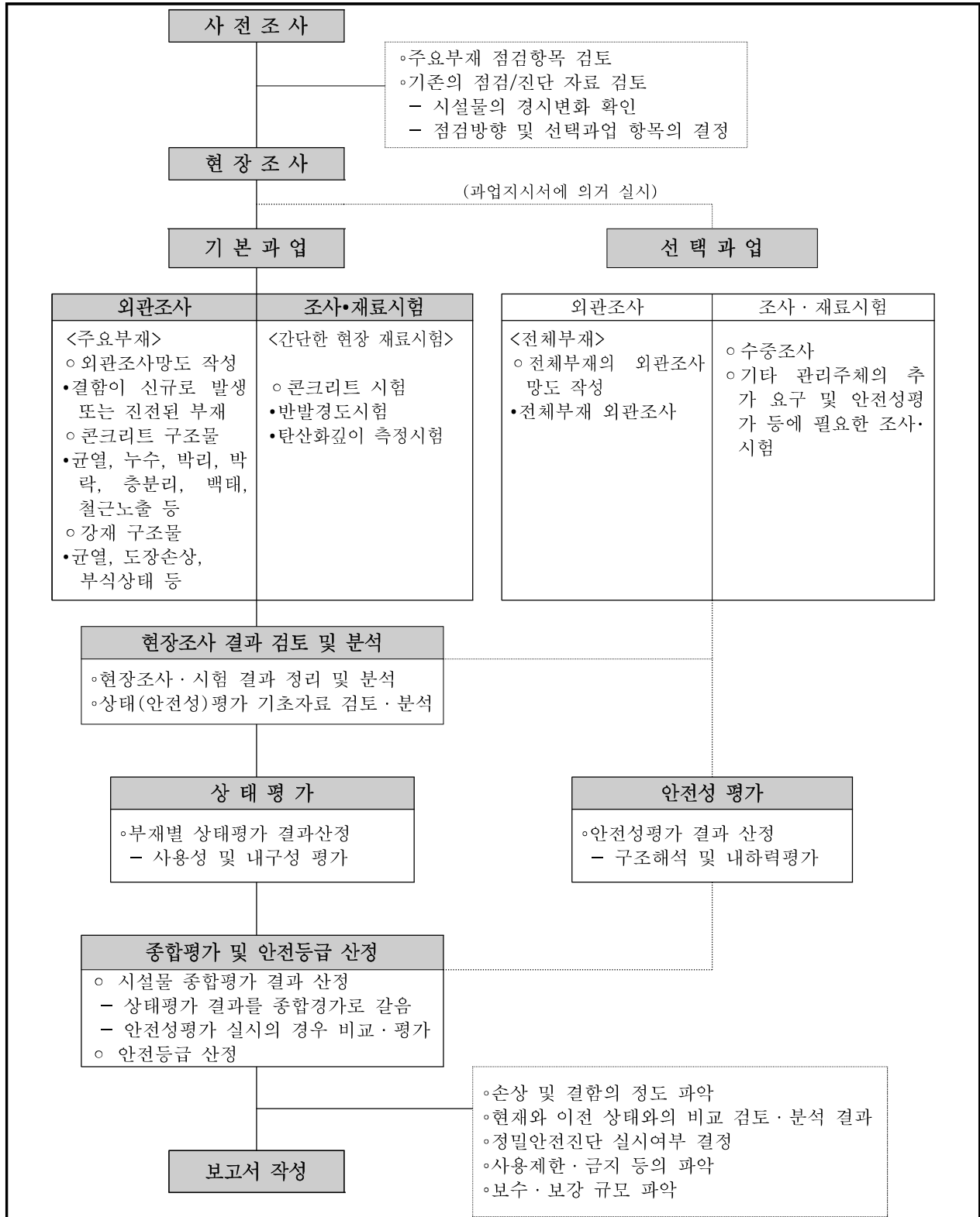
【그림 1.3.1】 교량 정밀안전점검 과업수행 흐름도
